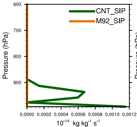
(e) non graupel IIC
