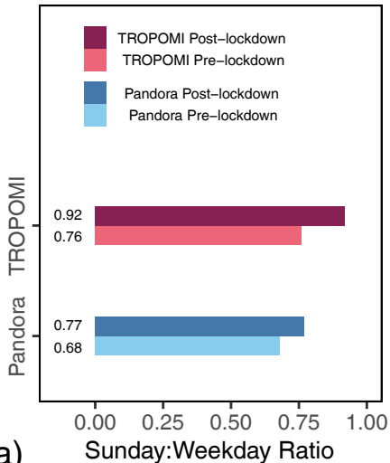
Pandora &amp; TROPOMI: Apr–Nov
