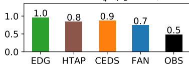
EANET: NH 4 + (μgN m -3 )
