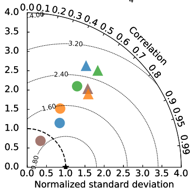
EANET: NH 4 + (μgN m -3 )
