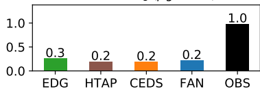
EANET: NH 3 (μgN m -3 )
