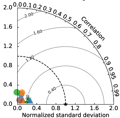
EANET: NH 3 (μgN m -3 )
