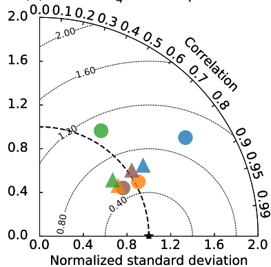
NTN: \text{NH}_4^+ wet deposition ( \text{gN m}^{-2} \text{yr}^{-1} )
