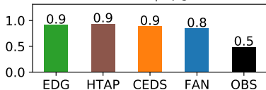
CASTNET: \text{NH}_4^+ ( \mu\text{gN m}^{-3} )
