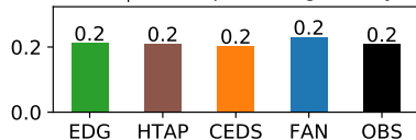
NTN: \text{NH}_4^+ wet deposition ( \text{gN m}^{-2} \text{yr}^{-1} )
