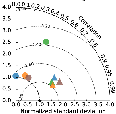
CASTNET: \text{NH}_4^+ ( \mu\text{gN m}^{-3} )
