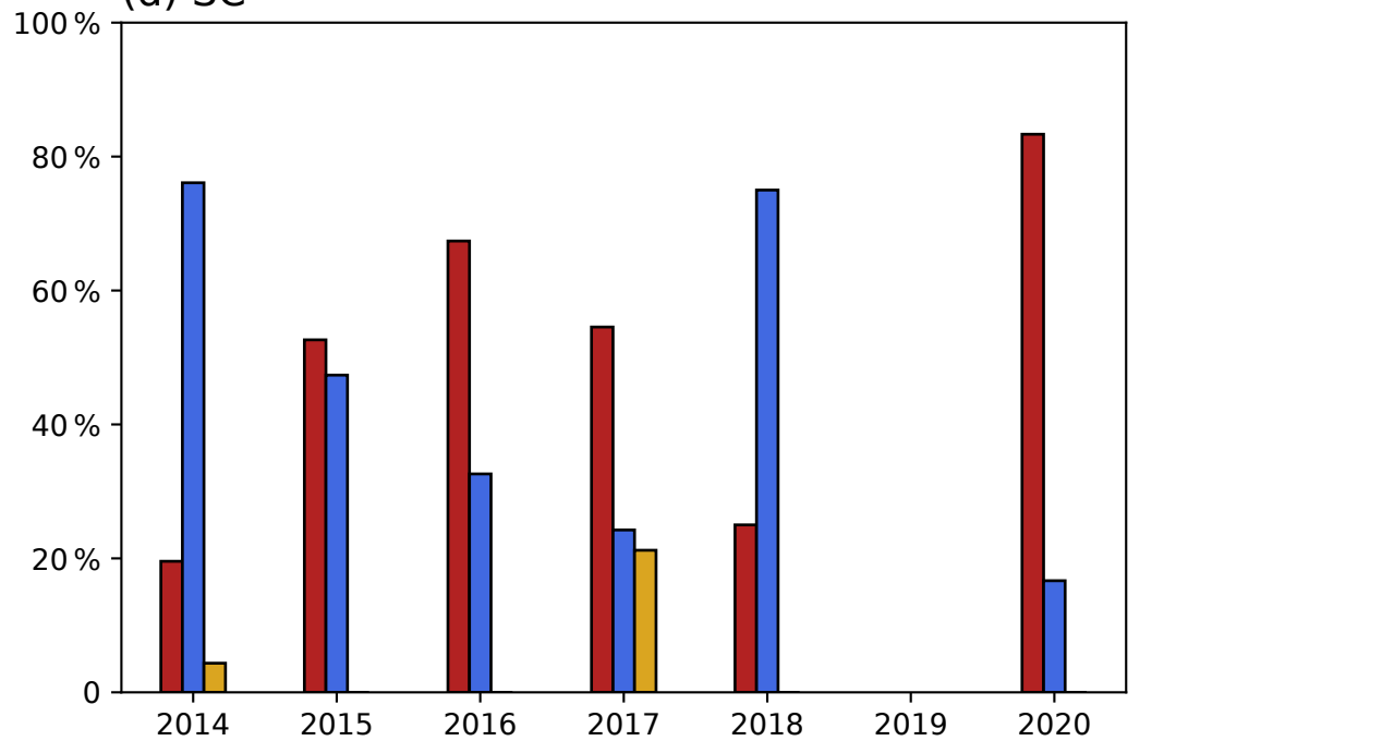
(d) SC
