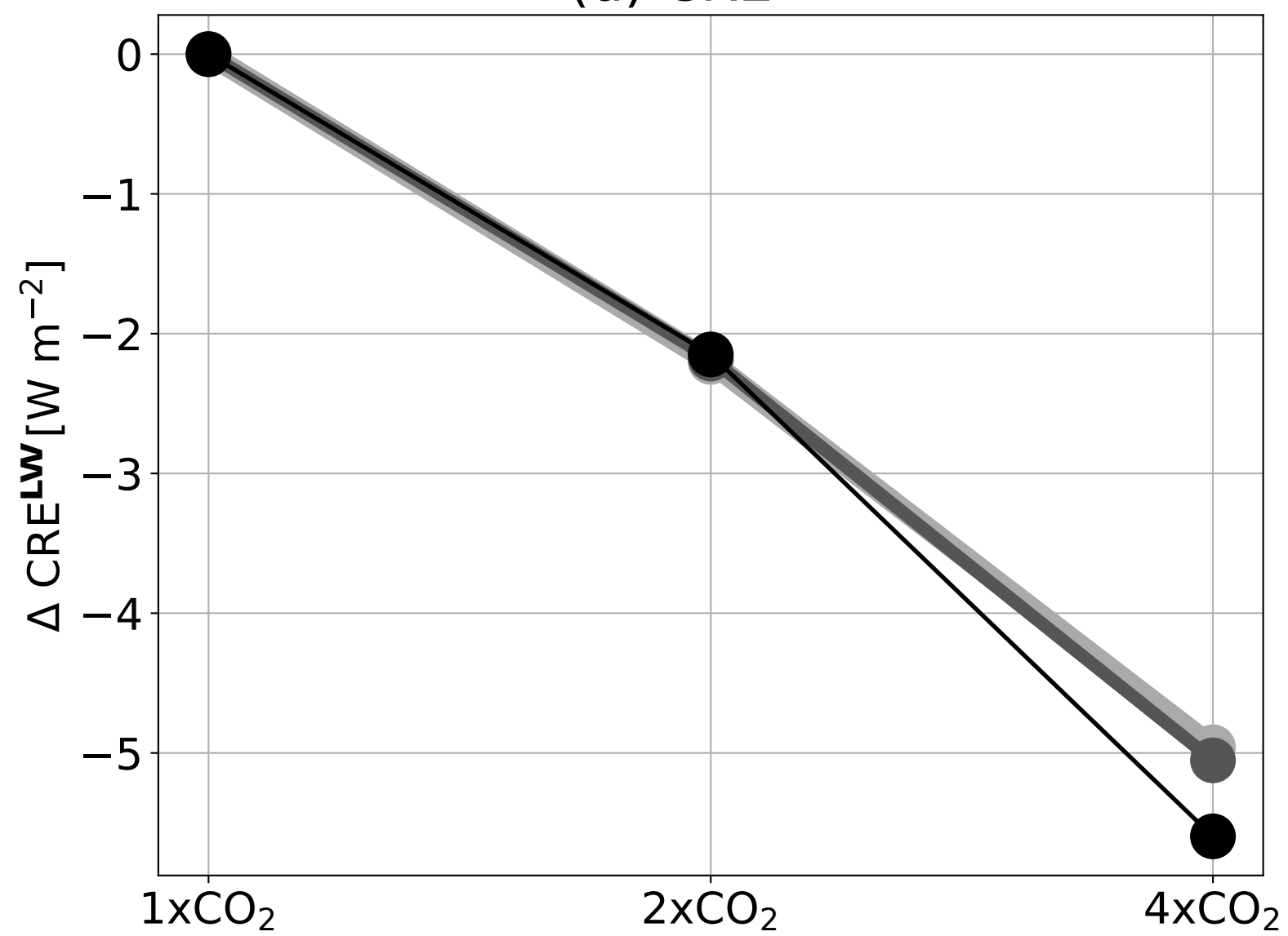
(d) CRE^{LW}
