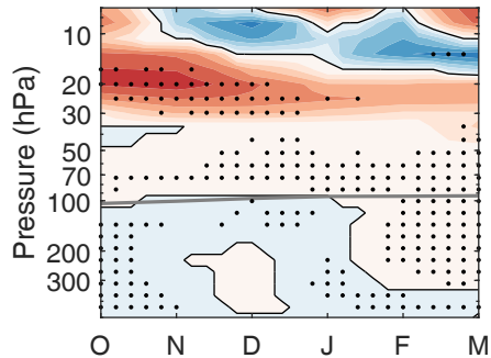
(g) CHM EP
