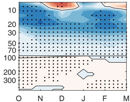
(i) CHM NIÑA
