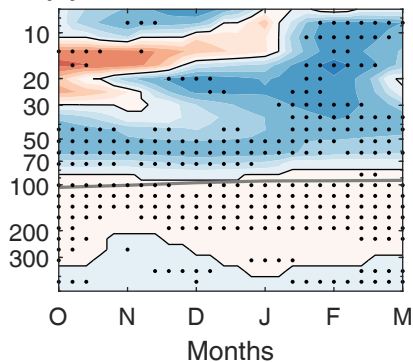
(h) CHM CP
