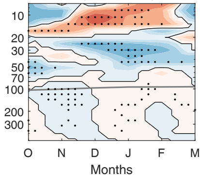
(e) ADV CP
