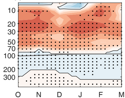
(f) ADV NIÑA
