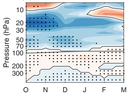
(d) ADV EP
