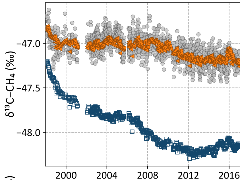
Tutuila (NOAA, American Samoa)
