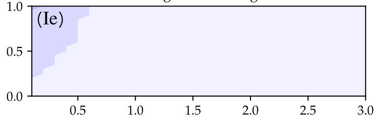
LUT: afglus - True: afglms
