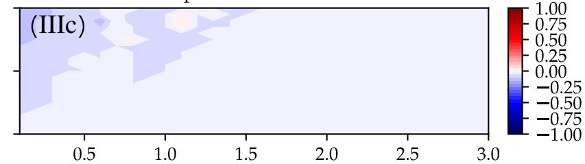
LUT: albedo 0.1 - True: albedo 0.2
