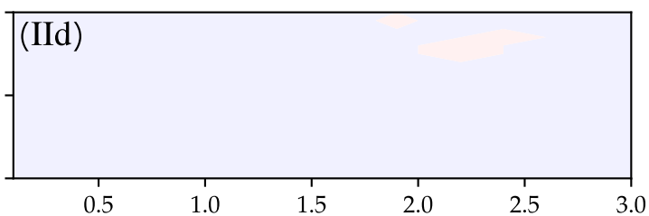
LUT: afglus - True: afglms
