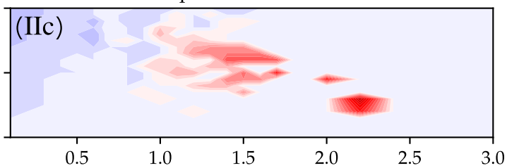
LUT: albedo 0.1 - True: albedo 0.2
