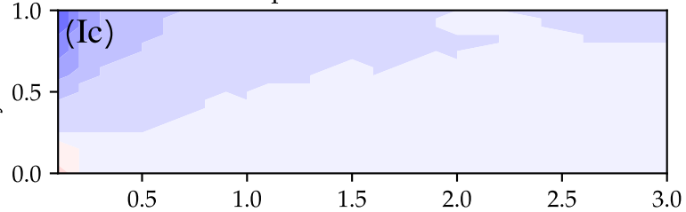
LUT: albedo 0.1 - True: albedo 0.2
