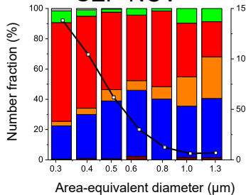
(g) SEP-NOV
