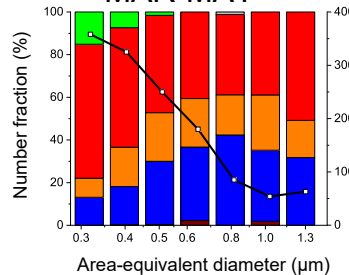
(e) MAR-MAY
