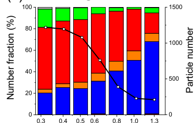
(d) DEC-FEB
