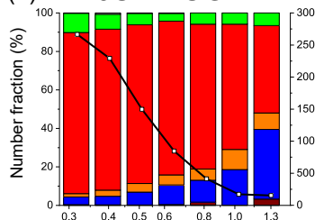
(b) JUN-AUG
