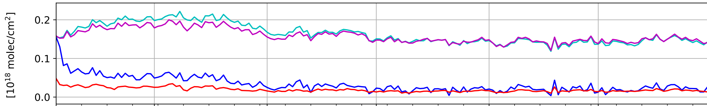
(b) IASI-B
