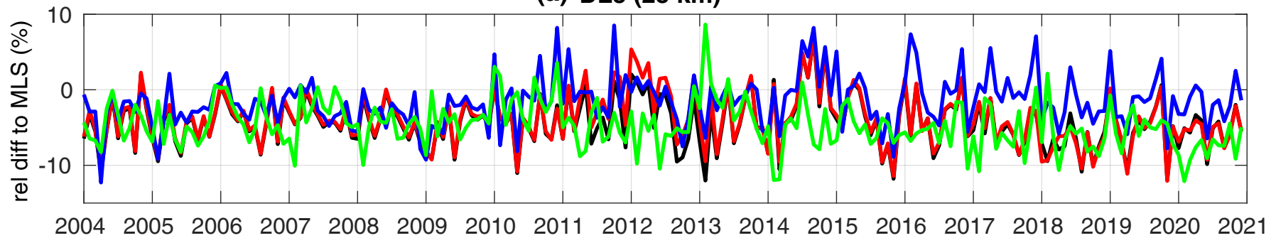
(b) DL8 (40 km)
