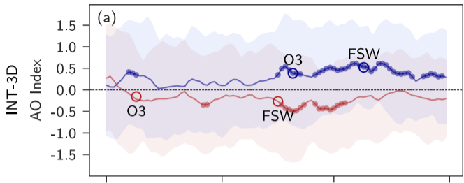
WACCM
