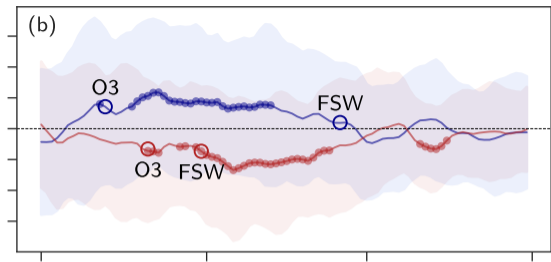
SOCOL-MPIOM
