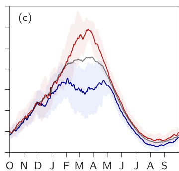
MERRA2
