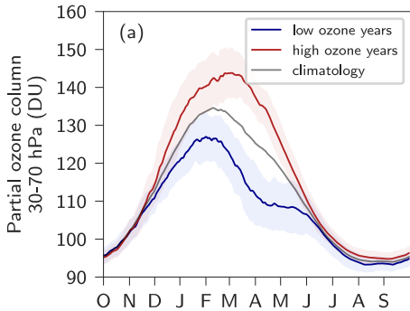
WACCM
