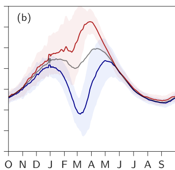
SOCOL-MPIOM
