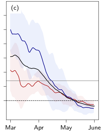
MERRA2
