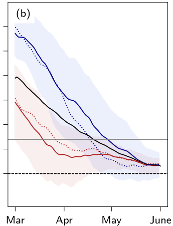
SOCOL-MPIOM
