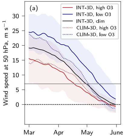
WACCM
