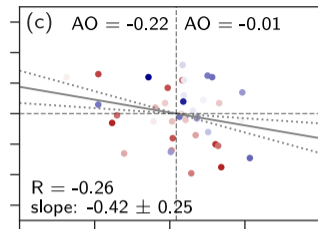
MERRA2
