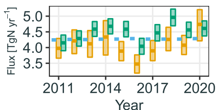
(d) Southern Hemisphere ( 90^{\circ} S – 30^{\circ} S)
