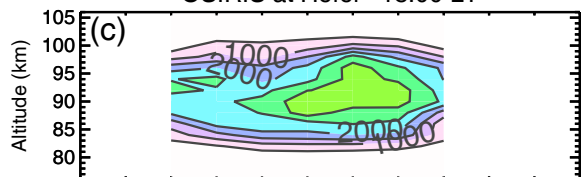
OSIRIS at Hefei ~18:00 LT
