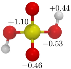
(a) \text{H}_2\text{SO}_4
