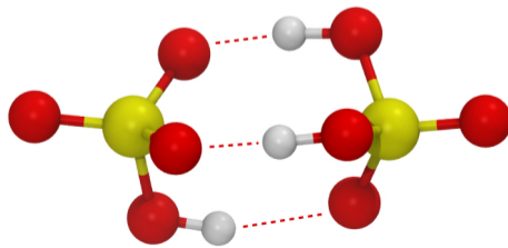
(g) [\text{H}_2\text{SO}_4 \cdot \text{HSO}_4^-]
