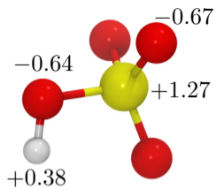
(b) \text{HSO}_4^-
