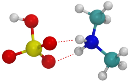
(f) [\text{HSO}_4^- \cdot (\text{CH}_3)_2\text{NH}_2^+]
