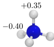
(d) \text{NH}_4^+
