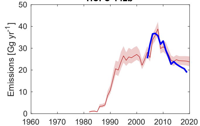
HCFC-142b
