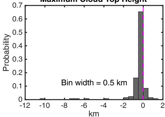
(d) rOn-2000 minus rOn-500 Maximum Cloud Top Height
