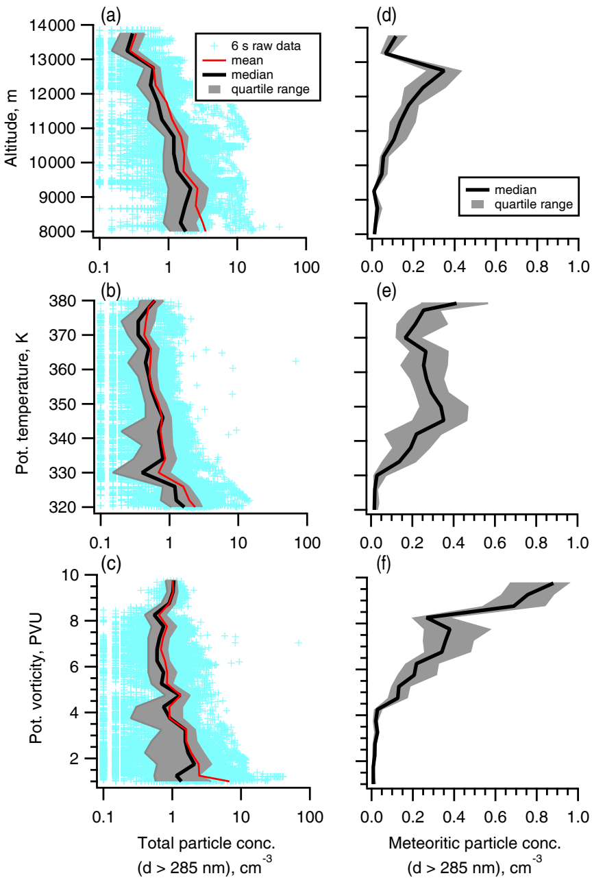
ML-CIRRUS 2014
