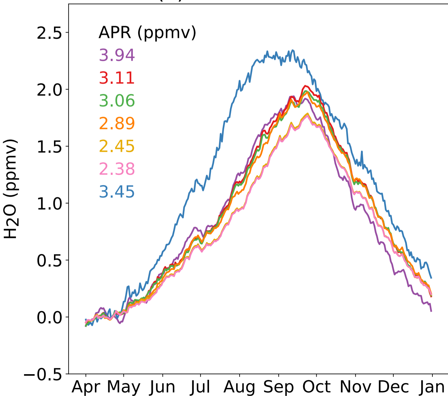
(d) NAMA at 100 hPa
