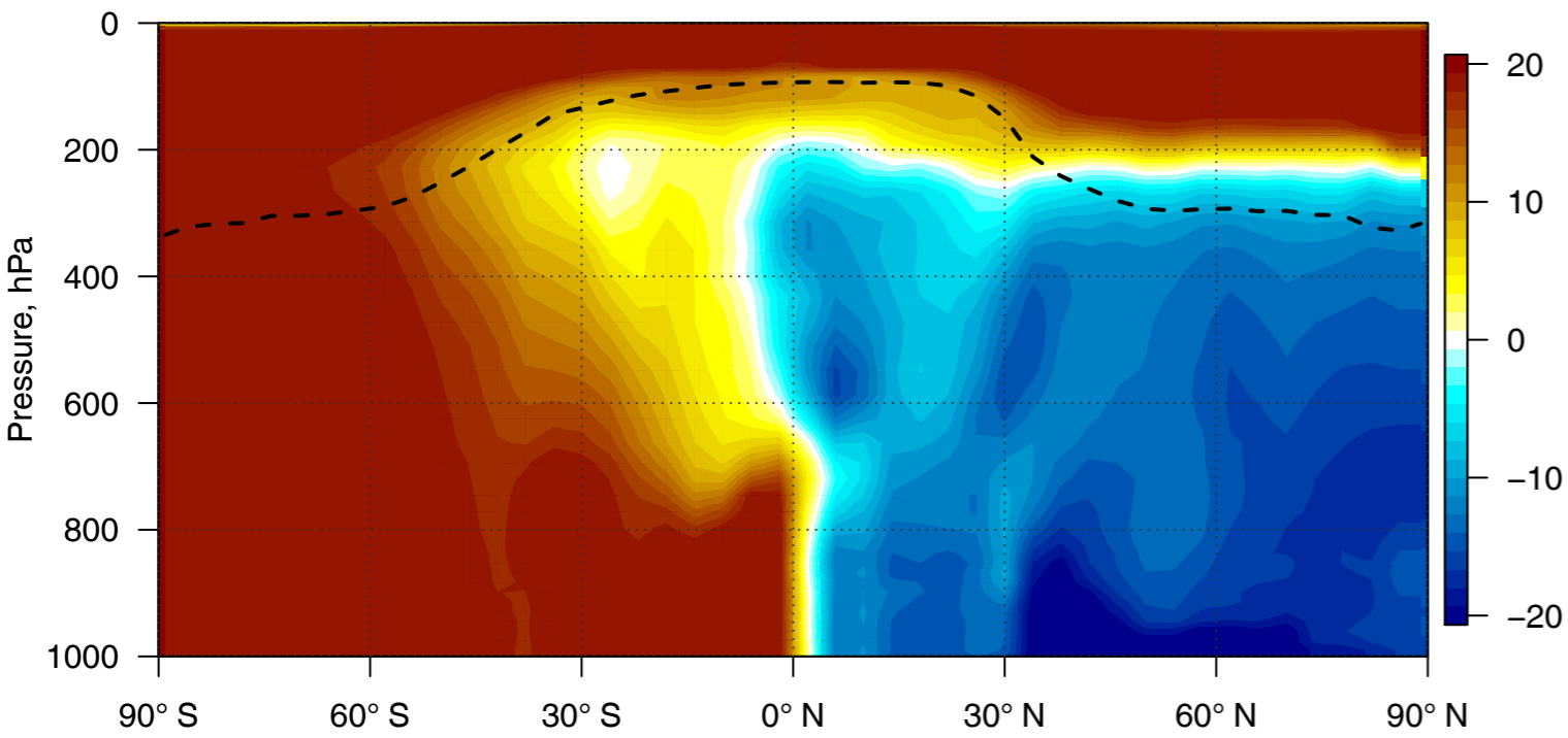
(a) CH 4 INI bias, 2010/02/01, [ppb]
