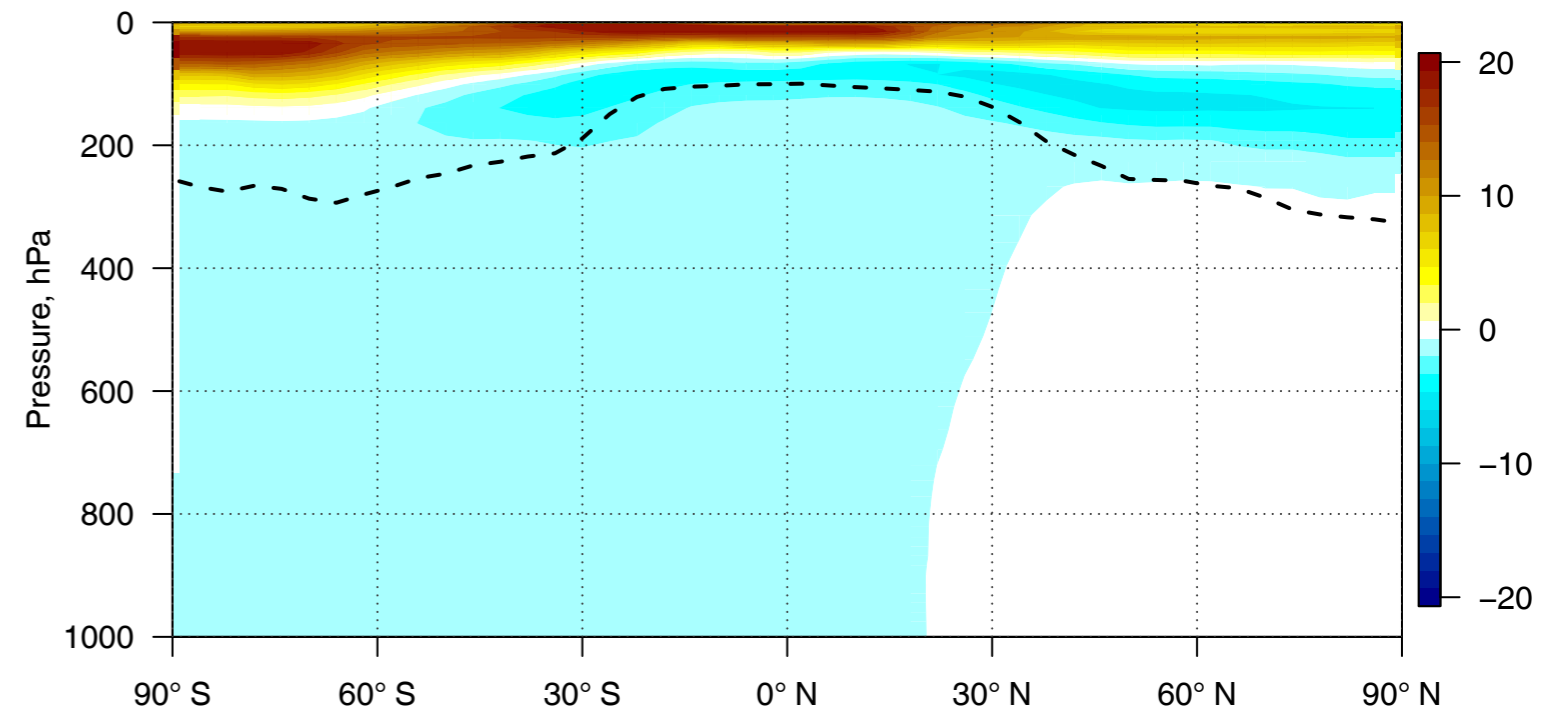
(b) CH 4 INI bias, 2010/05/31, [ppb]
