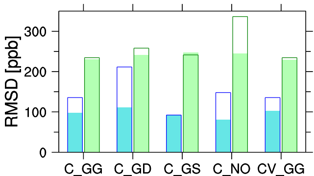
(d) CO
