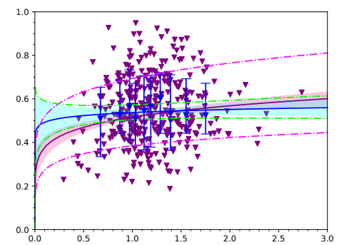
(12) Graupel
