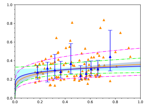
(6) Stellar
