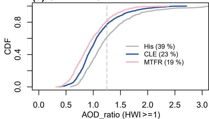
(d) GFDL-CM3
