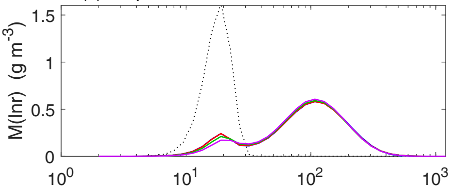
(d) droplet size distribution after 30 min
