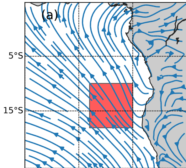
900 hPa (JJA)
