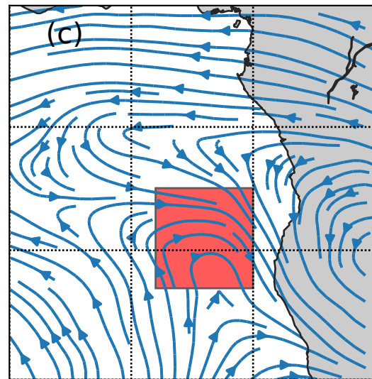
700 hPa (JJA)
