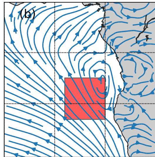
900 hPa (SO)
