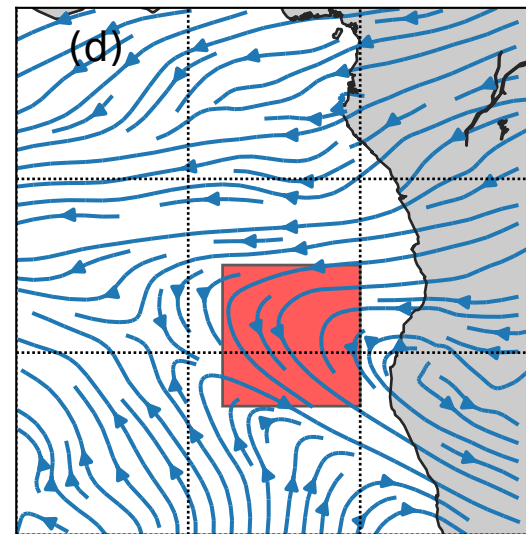
625 hPa (SO)
