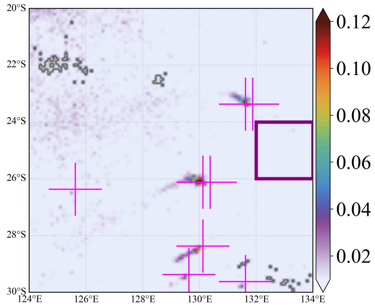
(b) XNO 2 [mmol m -2 ] 2018-12-23
