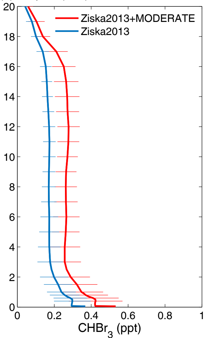
(b) Tropics (JJA)
