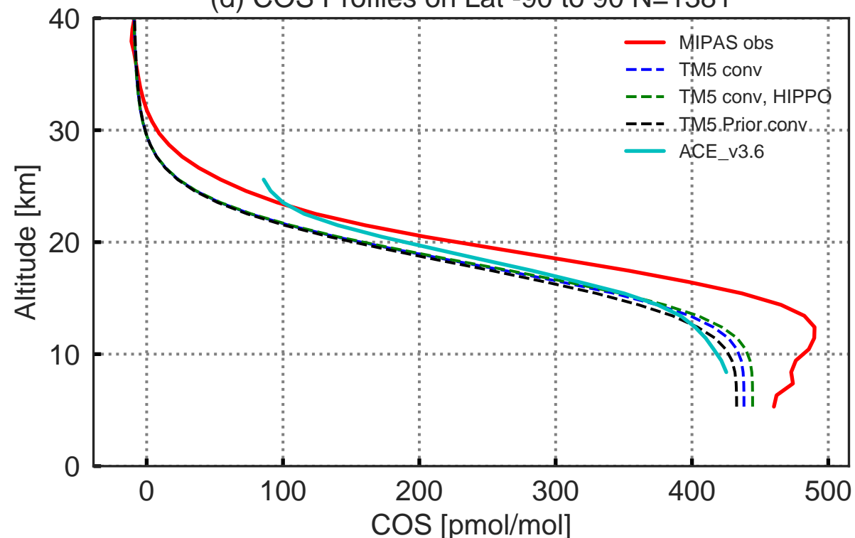
(d) COS Profiles on Lat -90 to 90 N=1381
