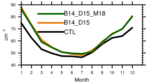
(d) CLDLLOW
