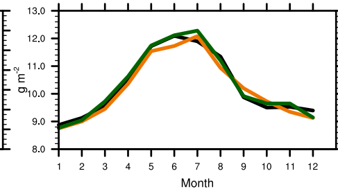
(h) IWP
