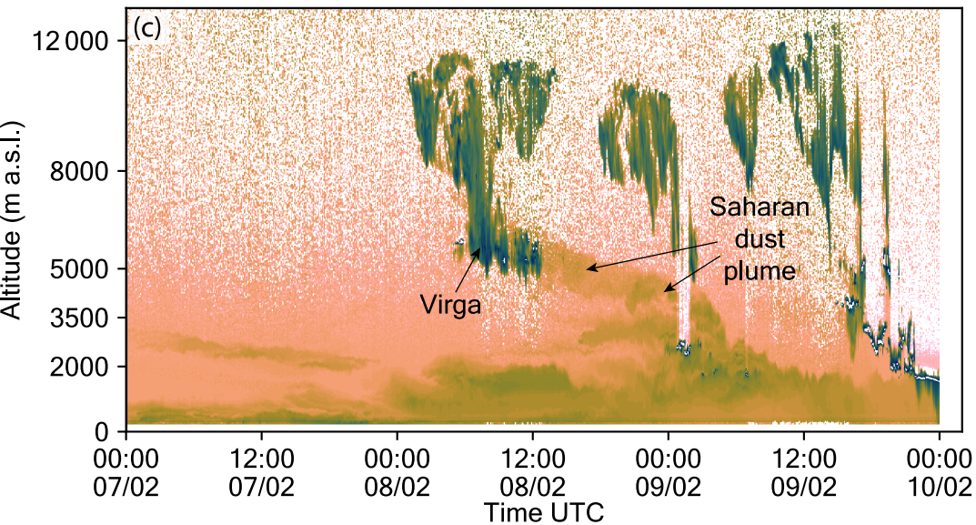
Ceilometer Freiburg 2020
