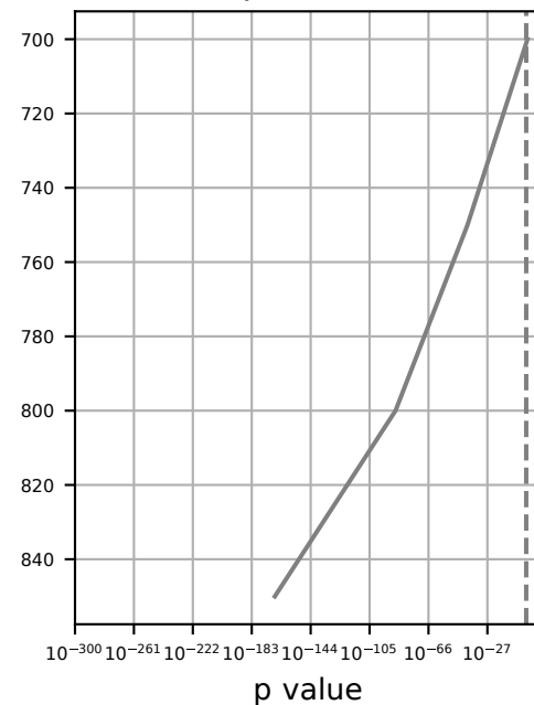
p value
