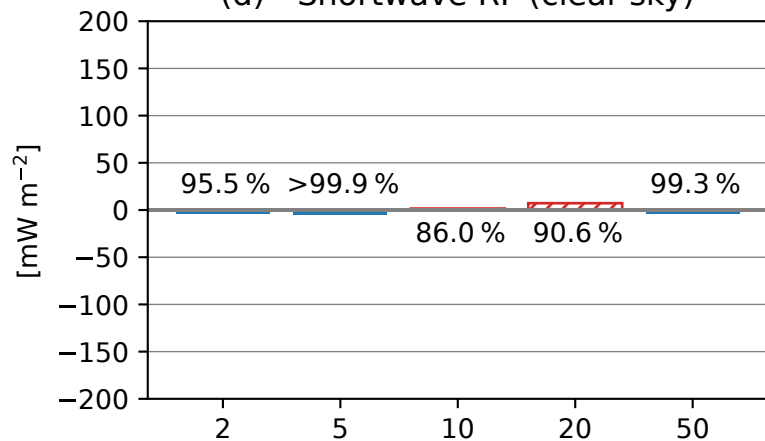
(d) - Shortwave RF (clear-sky)
