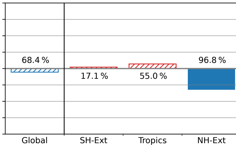
(b) - S_{\text{crit}}=1.3, f_{\text{act}}=10\%
