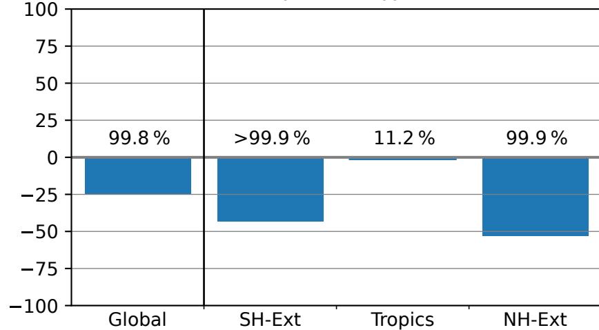
(d) - S_{\text{crit}}=1.2, f_{\text{act}}=1\%
