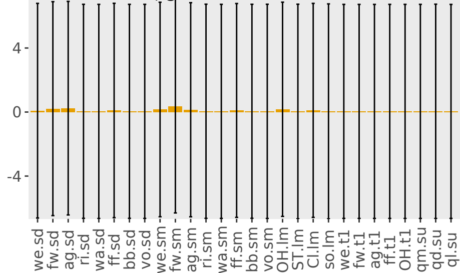
(d) \delta^{13}\text{C} - CH 4 inter-hemispheric difference
