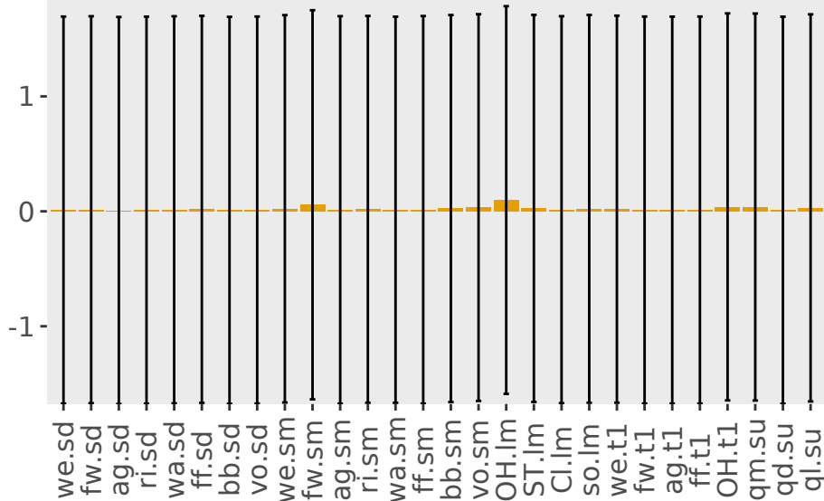
(e) CH 4 trend
