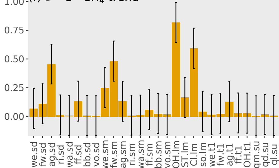
(f) \delta^{13}\text{C} - CH 4 trend
