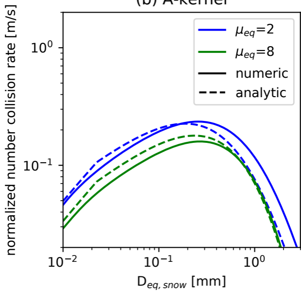
(b) A-kernel
