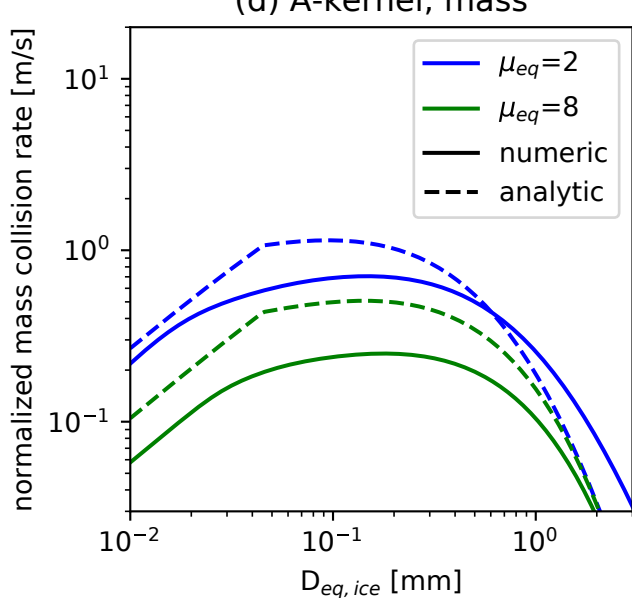
(d) A-kernel, mass
