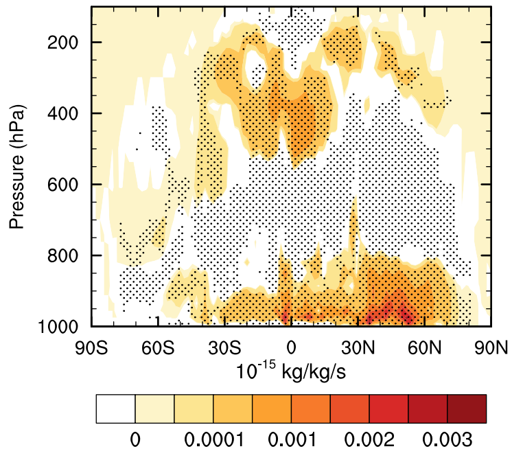
(b) Aitken: SOA
