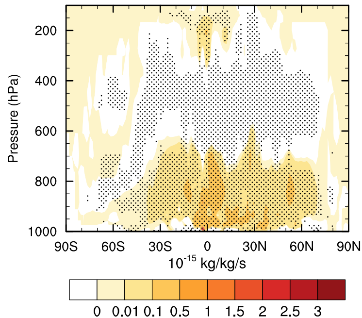
(d) Accumulation: POM
