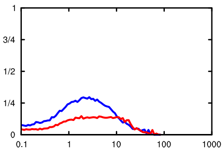
Coarse: Dust
