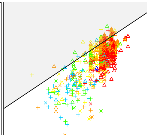
(d) NO x (2015)
