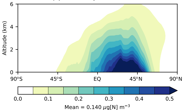
(d) FAST: \text{NO}_3 concentration
