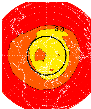
(d) Feb 1- NAVGEM
