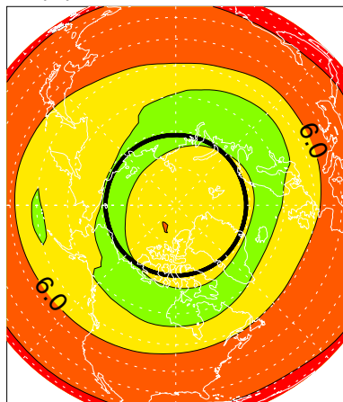
(d) Feb 1- NAVGEM
