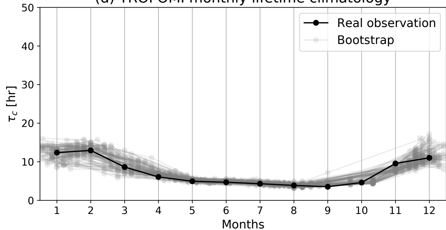
(d) TROPOMI monthly lifetime climatology
