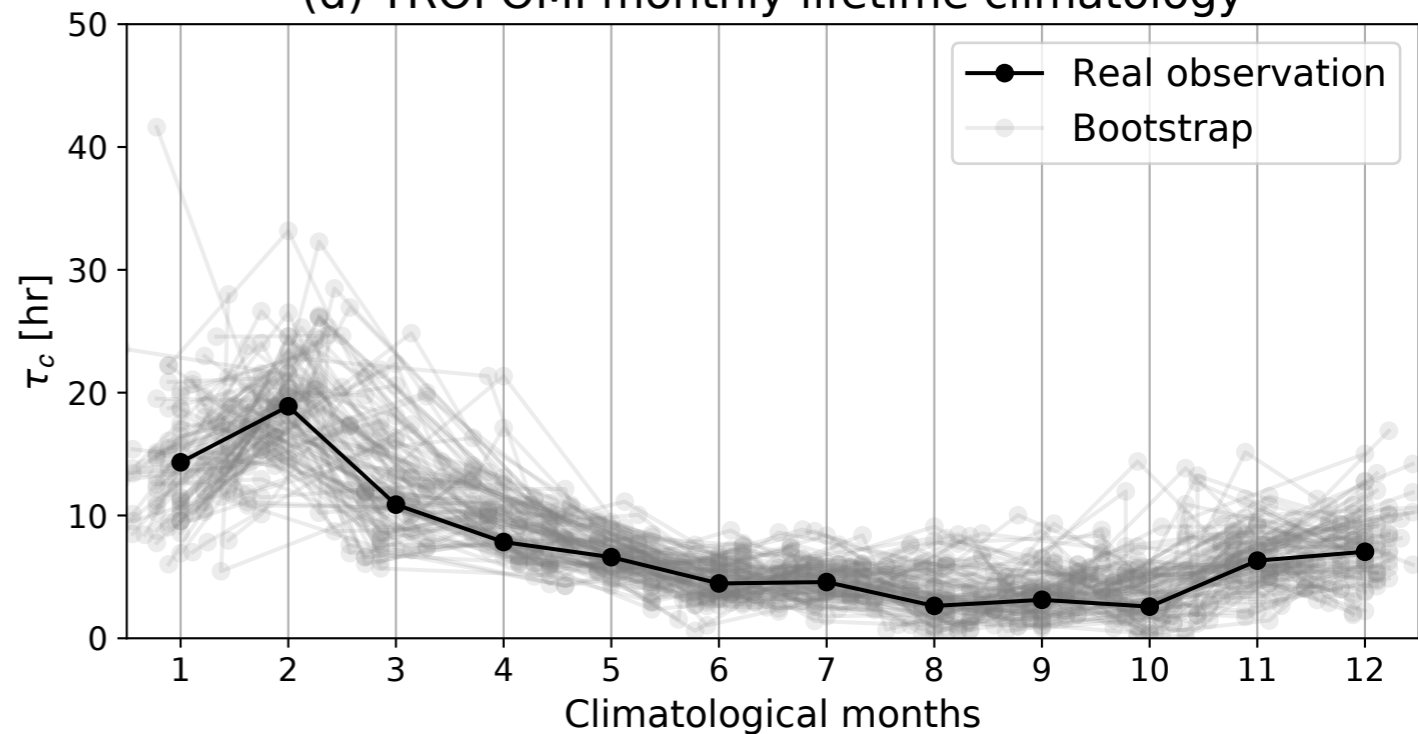
(d) TROPOMI monthly lifetime climatology
