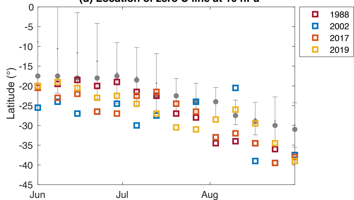
(d) Location of zero U line at 10 hPa
