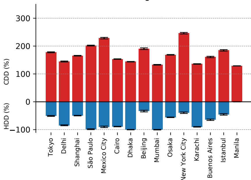
(d) CDD and HDD Change in 4.0 °C
