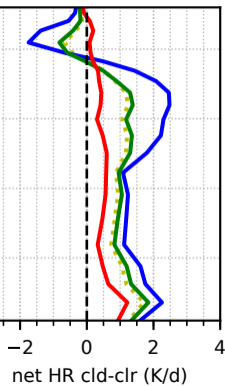
SST &lt; 300 K
