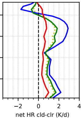
SST &gt; 302 K
